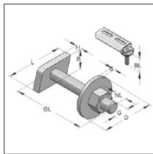
Śruba młotkowa z podkładką i nakrętką
